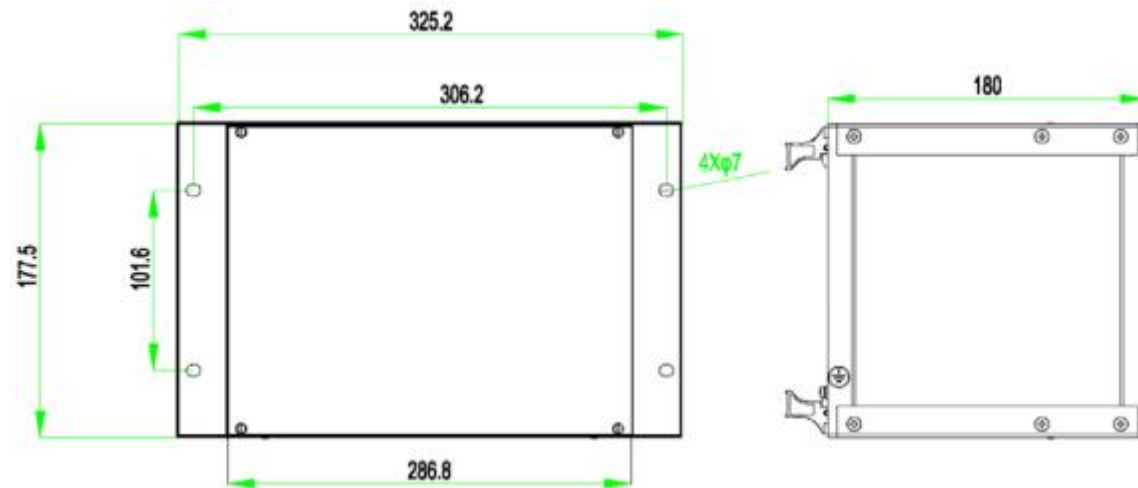
图 5-3 本体正面、侧面视图(单位: mm)
