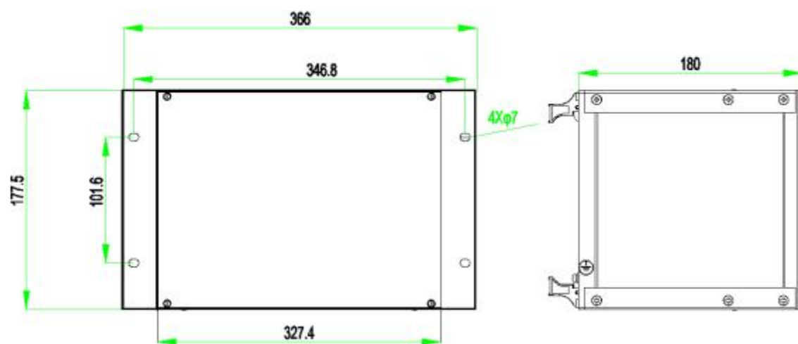
图 5-4 本体正面、侧面视图(单位: mm)
