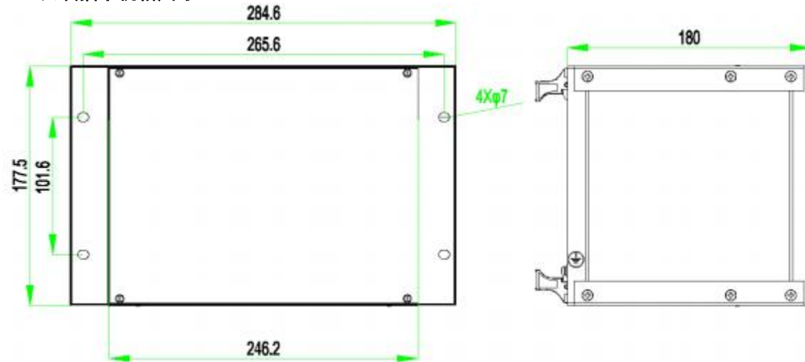
图 5-2 本体正面、侧面视图(单位: mm)
